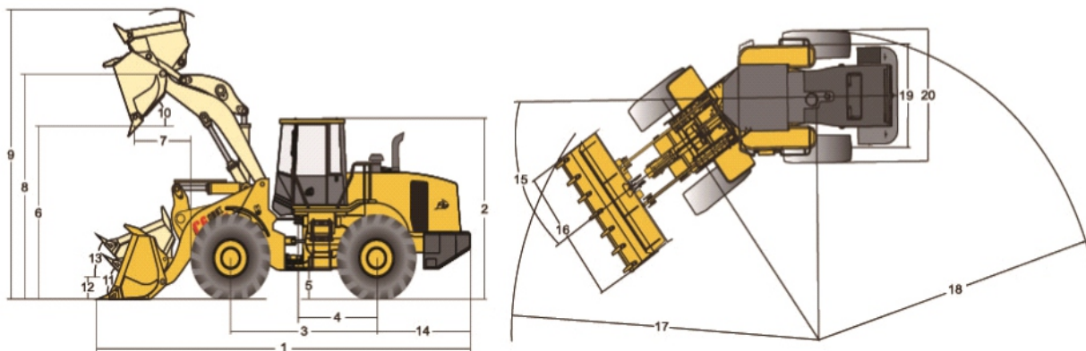
整机外形尺寸 (长×宽×高) 8500×3130×3550mm
